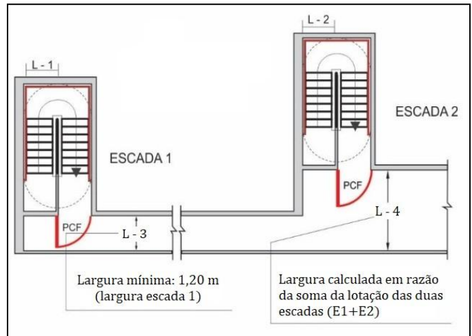
Figura 26: Dimensionamento de corredores de descarga.
