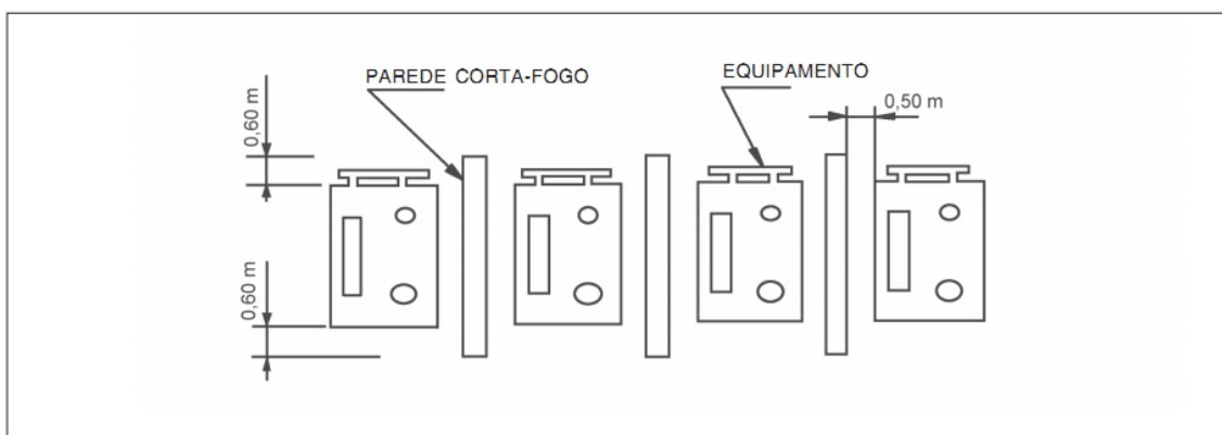
Figura 3: Separação por parede corta-fogo entre equipamentos
