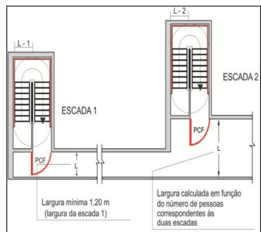
Figura 19 - Dimensionamento de corredores de descarga
