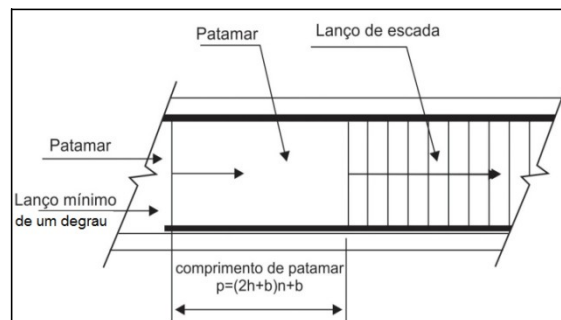
Figura 6 - Lance mínimo e comprimento de patamar
