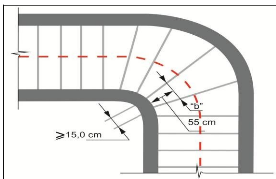
Figura 5 - Escada com lances curvos e degraus balanceados
