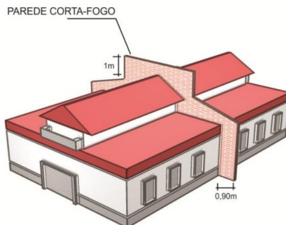
Figura 8: Parede corta-fogo
