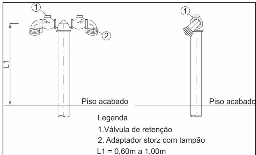
II – DISPOSITIVO DE RECALQUE TIPO COLUNA
