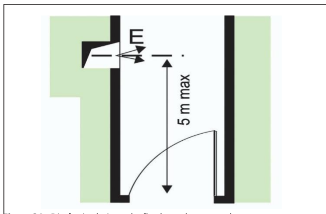
Figura 24: Distância de introdução de ar de portas de acesso
