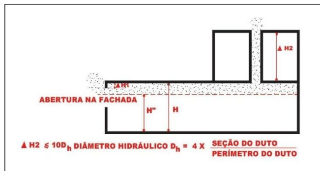
Figura 16: Diâmetro hidráulico
