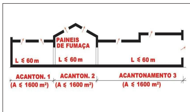
Figura 12: Divisão em áreas de acantonamento
