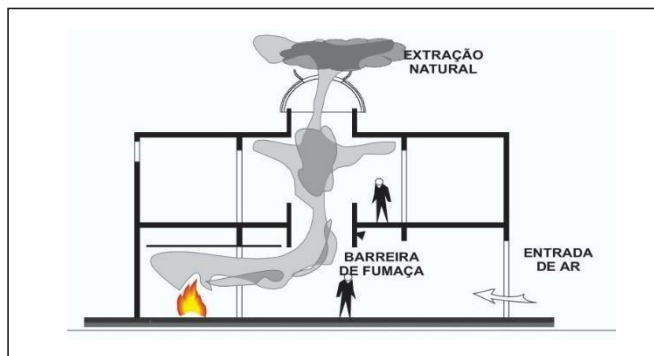
Figura 10: Exemplo de controle de fumaça por extração natural e entrada de ar natural, diretamente
