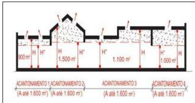
Figura 15: Altura de referência diversificada por acantonamento
