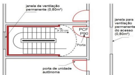
Figura 15: Ventilação da escada enclausurada protegida e seu acesso.
