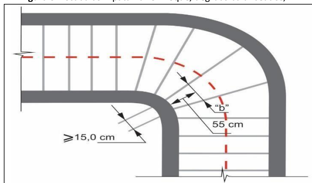
Figura 6: Escada com patamar em leque, degraus balanceados,
