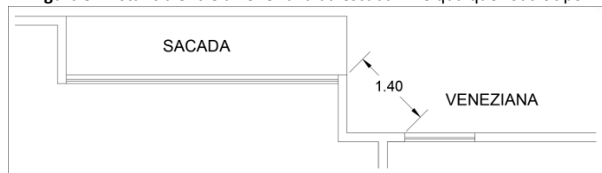
Figura 9: Distância entre a veneziana da escada EP e qualquer outro tipo de
