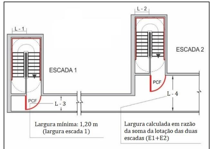
Figura 26: Dimensionamento de corredores de descarga.
